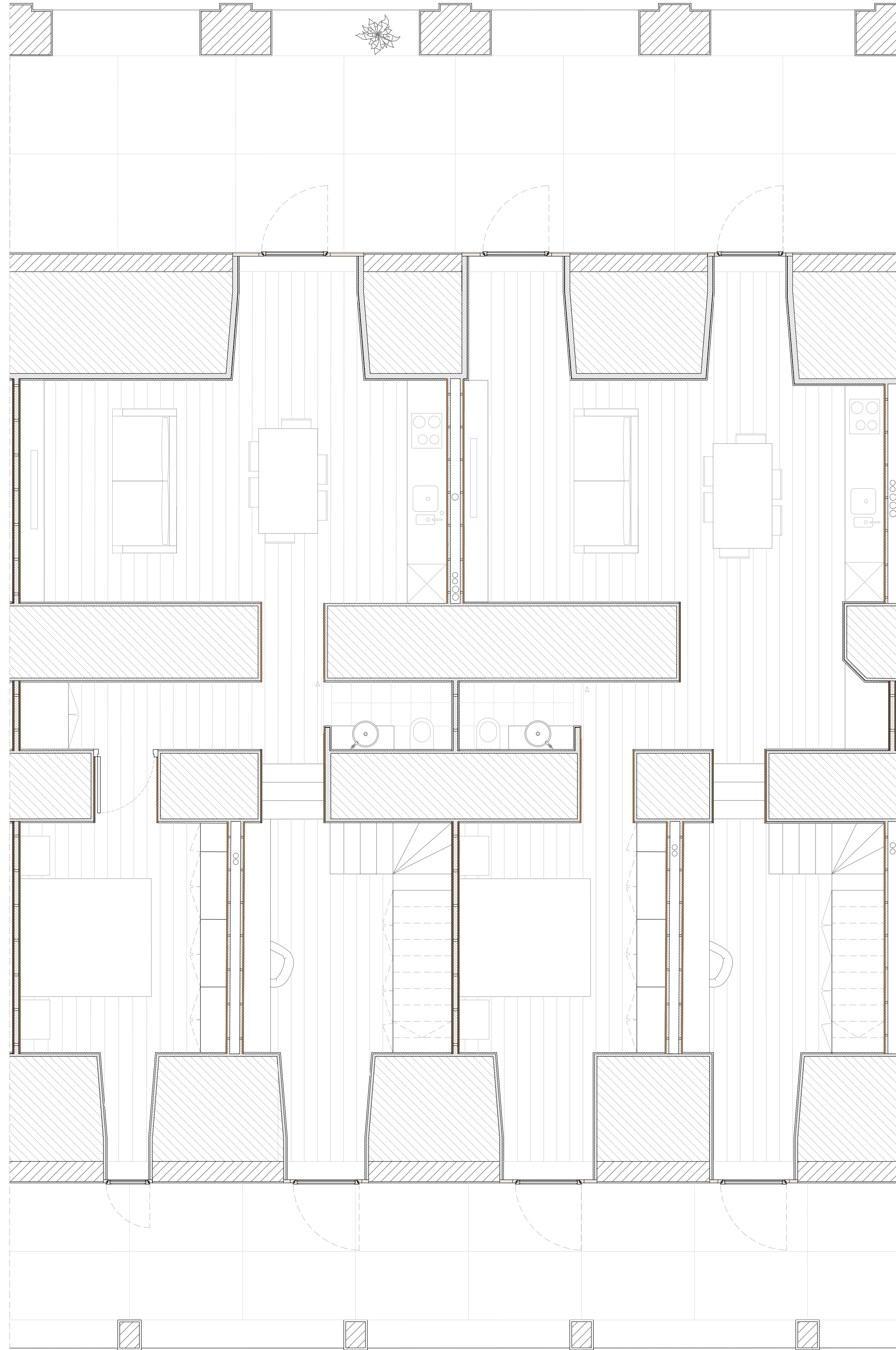
PISO 0
